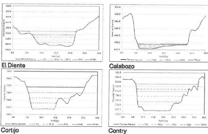
Figura 6. Nivel del río por sitio para diferentes eventos de precipitación con diferentes periodos de retorno. Elaboración propia.
